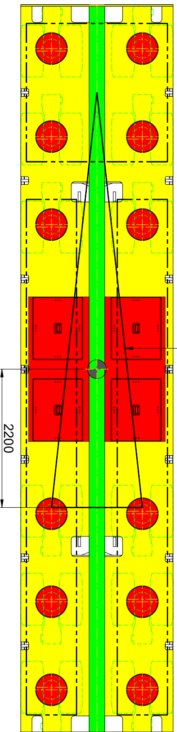
Triangolo di stabilità / Stability triangle
